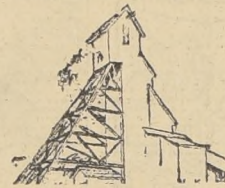
El fondo de las minas Kolar, en la India, es tan ardiente y las presiones son tan tremendas, que la roca esquistosa impregnada de oro fluye como plástica moldeable.
