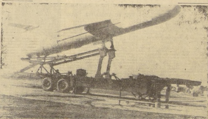
EL PASO (Texas).— La Fuerza Aérea norteamericana anunció el 7 de febrero que se realizó con éxito un vuelo de prueba del proyectil táctico "M-70-MACE", usando un nuevo sistema de control colocado a bordo. El "MACE" fue lanzado desde el centro de desarrollo de proyectiles de la Fuerza Aérea, cerca de Alamo Gordo, Nuevo México. — (RADIOFOTO DE LA UNITED PRESS)
