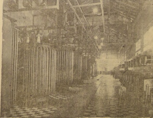
Una Sección de la Sub Estación Eléctrica de la Fábrica de "Cemento el Melón", en La Calera.
