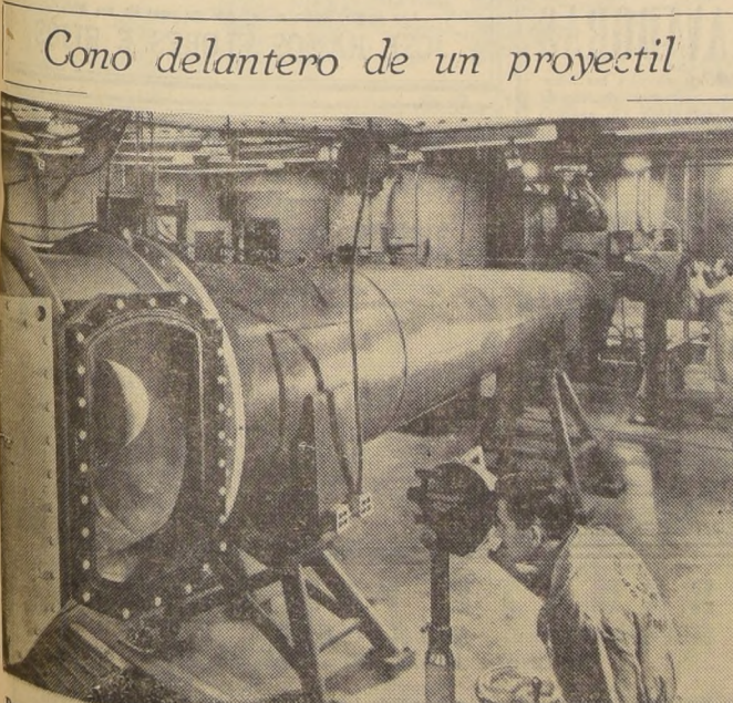
Cono delantero de un proyectil. Este túnel, capaz de reproducir velocidades de 32.400 millas por hora, se utiliza para estudiar las velocidades requeridas para colocar vehículos en órbitas alrededor de la Tierra, y para asegurar sus reentradas a la atmósfera terrestre.
