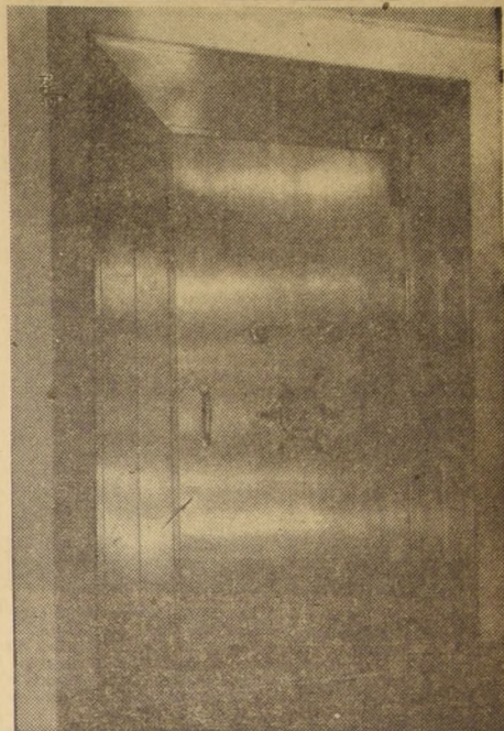
PUERTA BLINDADA DE ACERO INOXIDABLE. — La puerta que ilustra el presente grabado está colocada en la bóveda del Tesoro del Banco. Su peso es de varias toneladas. Se cierra sin llaves, solo con dos cerraduras de combinación con cien millones de diferentes claves. Construida de acuerdo a un moderno diseño y totalmente en acero inoxidable, esta obra se realiza por primera vez enteramente en el país por la firma Cajas Bash Sociedad Industrial Limitada.
