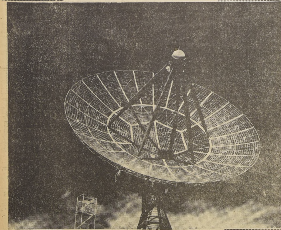
DEBUTO RECIENTE.— Esta antena de radar en forma de plato y de 60 pies de diámetro, que se encuentra ubicada en la Base Vandenberg, de la Fuerza Aérea de los Estados Unidos, en California, fue la primera en registrar el rumbo que seguían el satélite Descubridor I, y su vehículo Thor, de propulsión, después de haber sido lanzados desde esa misma base. Es parte de una completa red de estaciones localizadoras y de telemetría que se extienden desde la costa del Pacífico hacia el Occiden-
