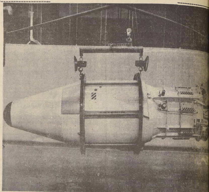
ANTES DE LA PARTIDA.— Este es el "Descubridor I", el noveno satélite lanzado por los Estados Unidos, el que quedó colocado en una órbita polar. El Descubridor I, fue lanzado por la Fuerza Aérea de los Estados Unidos desde sus instalaciones para el ensayo de proyectiles balísticos en la costa occidental, en la Base Vandenberg, California. Impulsado hacia su órbita por un proyectil balístico de alcance intermedio Thor, que sirvió como etapa inicial de propulsión, el "Descubridor" recibe su
