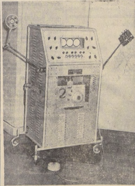
Equipo de electromiografía Micoathograph Alvar.
