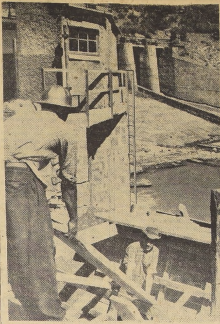
LUCHA CONTRA LA NATURALEZA. - Un aspecto de la bocatoma de la Planta de Quelchues, que fue virtualmente "estrujada" por uno de los cerros que se deslizo 50 centímetros, destruyendo las obras de esta importante instalación.
