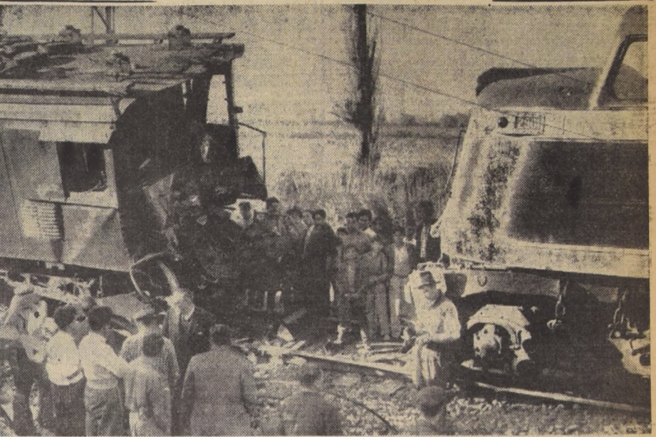
EL GRAFICO evidencia la magnitud del choque de la locomotora 2101 que conducía el tren N.º 8, de pasajeros, de Santiago a Valparaíso y la máquina 2101 (venía de Llay-Llay a Santiago). La colisión se produjo en las cercanías de Quilicura. La violencia del impacto destruyó casi por completo la parte delantera de la locomotora 2101. Su conductor, Ignacio Moraga (17 años de servicios), quedó gravemente herido. Fue internado en el Hospital José Joaquín Aguirre.
