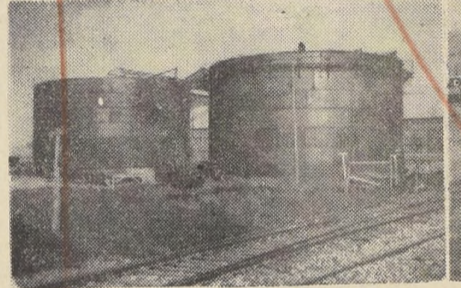
El grabado muestra tres aspectos de los sólidos y enormes estanques para la melaza, montados por "Ward, Della Maggiora y Cia. Ltda.", en la planta azucarera de Linares. Estos trabajos, de gran precisión y seguridad, confirman la jerarquía técnica de la prestigiosa firma.
