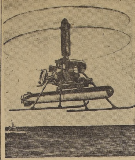
WASHINGTON.— Este es el DSN-1 Drone, el helicóptero mator de submarinos. Es un dibujo de lo que se construye actualmente en la Gyrridyns Company of America, Inc., en St. James, Long Island, por orden de la Armada norteamericana. Este helicóptero es guiado por control remoto. El primer destructor que lleve esta nueva arma, será el Hazelwood. (Foto UPI)
