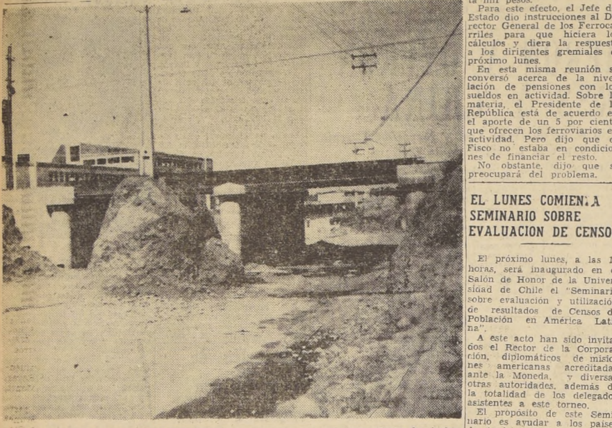
FASO BAJO NIVEL EN "LO VALLEDOR" — Se encuentran en sus fases finales los trabajos de terminación del paso bajo nivel de la vía, construido por la Empresa de FF. CC. del Estado, en San Joaquín, al llegar al Matadero "Lo Valledor". Esta nueva ruta descongestionará el tránsito de vehículos por la Avenida Pedro Aguirre Cerda, y el empalme al camino a Melipilla. Tendrá dos calzadas de 7 metros. La Oficina de Vialidad, hizo el movimiento de tierra para los accesos con un total de nueve mil metros cúbicos. Los trabajos de pavimentación se iniciarán tan pronto la Compañía Chilena de Electricidad cambie la postación de alta tensión. Podrá ser entregado al tránsito público dentro de los setenta días. Los trabajos ejecutados por Vialidad, tienen un costo del orden de los sesenta millones de pesos. Este paso también dará salida a la Carretera Panamericana, de la cual dista doscientos metros.
