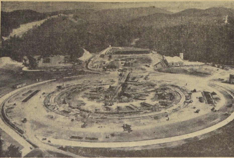
EE. UU. CONSTRUYE EL MAYOR RADIOTELESCOPIO DEL MUNDO. — Los cimientos del mayor radiotelescopio del mundo, en su terreno de unos 1.500 acres de extensión, en planas montañas de Virginia. La estación, construida bajo el programa de la división naval de la Armada, tiene un costo de 79 millones de dólares y permitirá a los científicos sintonizar señales de radio desde cuerpos astrales situados a 38 millones de años luz de distancia.
