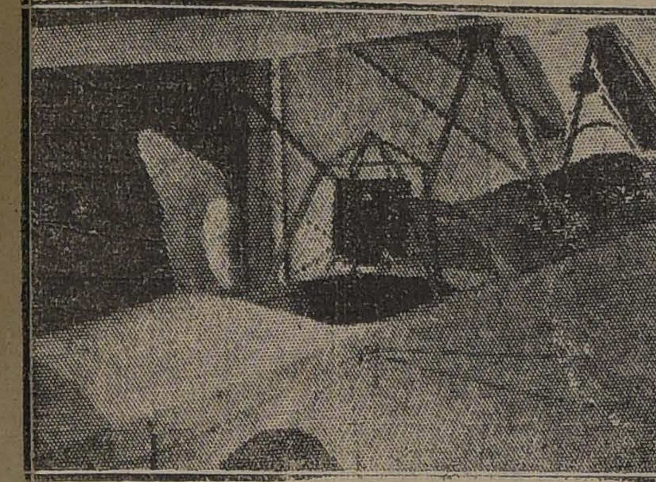
Disposiciones de los instrumentos meteorológicos en un avión destinado a investigaciones aerológicas
