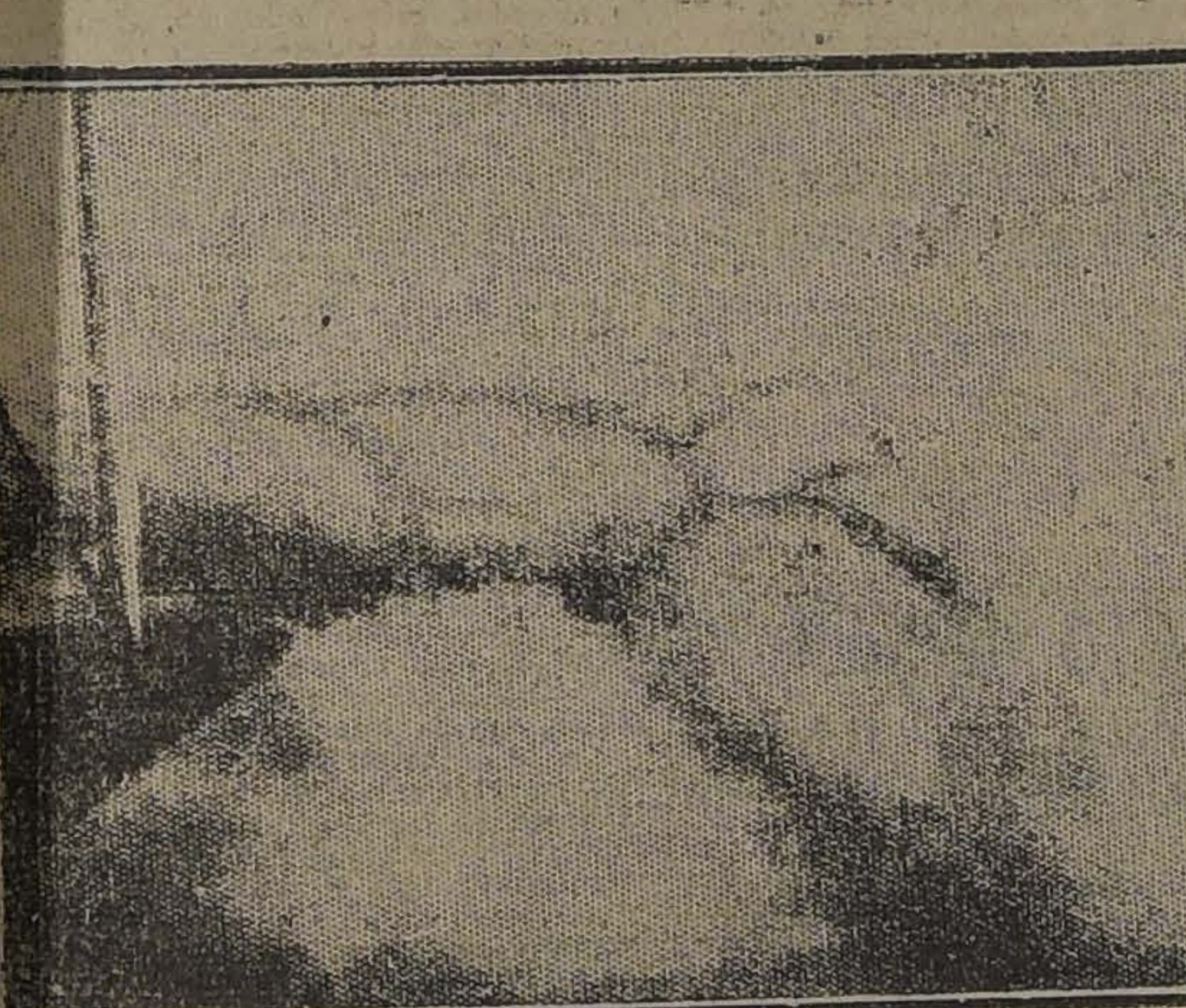
Mar de nubes fotografiado desde un avión cumulus-stratus
