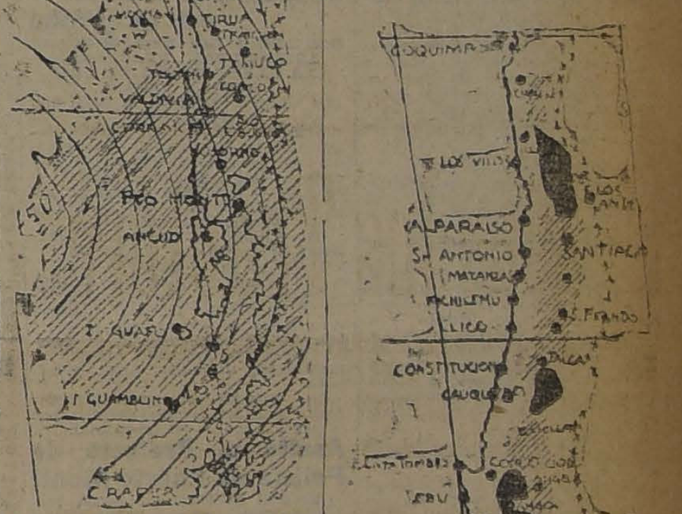
LA DEPRESION QUE ORIGINO LOS MALOS TIEMPOS DEL 7 Y 8 EN LA ZONA SUR
