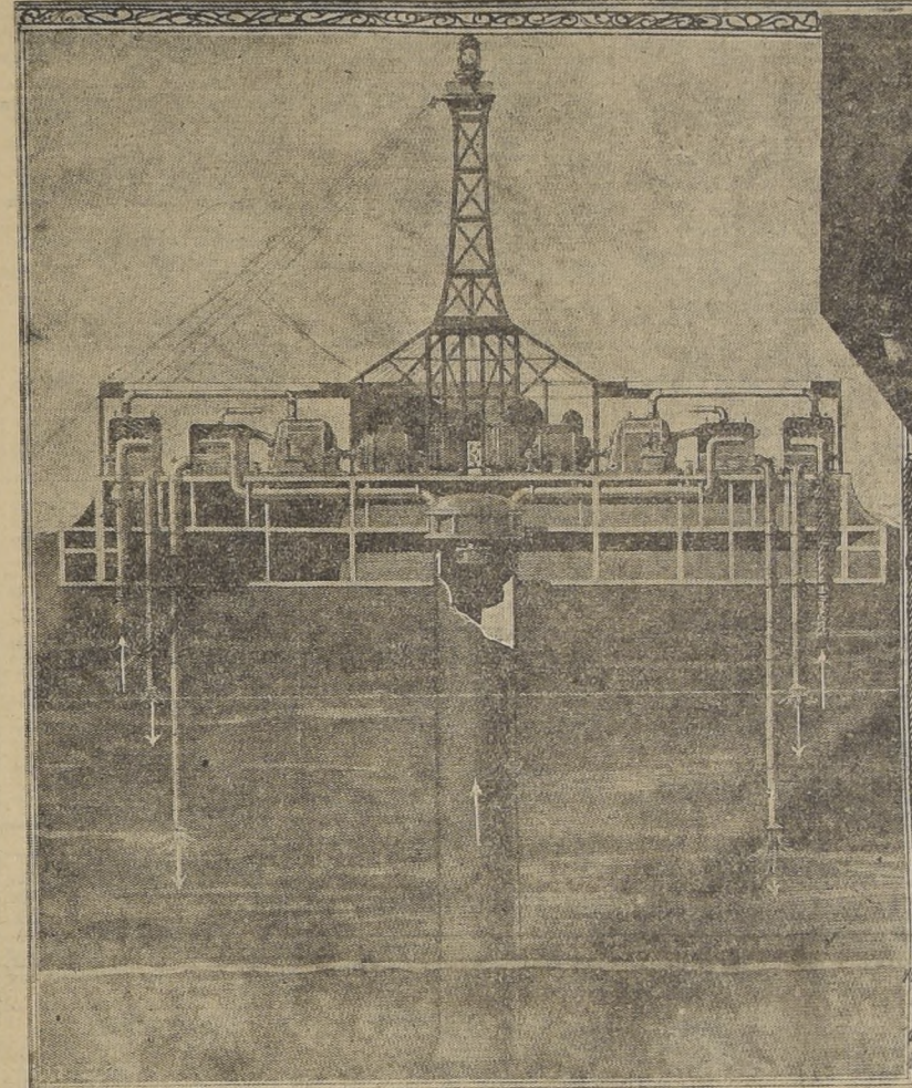
Una Usina Hidro-Térmica en el Océano, según los planos de MM. Claude y Boucherot — M. George Claude — El aparato en que MM. Claude y Boucherot han realizado sus experiencias
