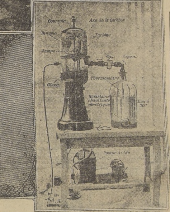
El aparato en que MM. Claude y Boucherot han realizado sus experiencias
