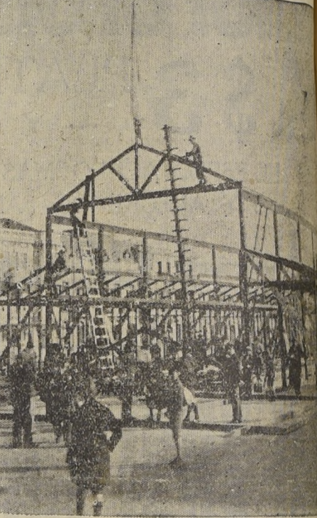
El primer tijeral levantado ayer en el pabellón que se construye para la Exposición de Paños de la Sociedad Nacional de Paños de Tomé
