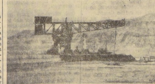
LA GRUA TITAN PARA FABRICAR BARCOS — En este lugar del puerto de Iquique se instalarán los asilleros que producirán hasta dos embarcaciones mensuales. La grúa se instaló en el grabado, servirá para sujetar el casco y demás instalaciones hasta un peso total de setenta toneladas. Luego se harán las terminaciones en el agua. Doscientos obreros tendrán ocupación en esta faena. (Foto de José Herrera.)
