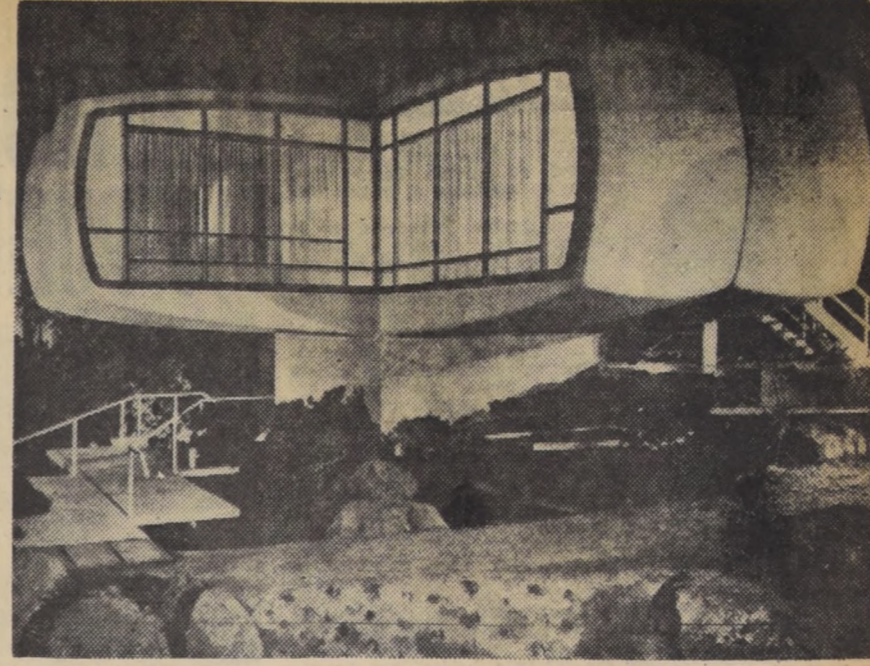
Sobre un núcleo cuadrado, de 16 pies de lado, se extiende en voladizo la casa construida en materiales plásticos que se encuentra en Disneylandia.
