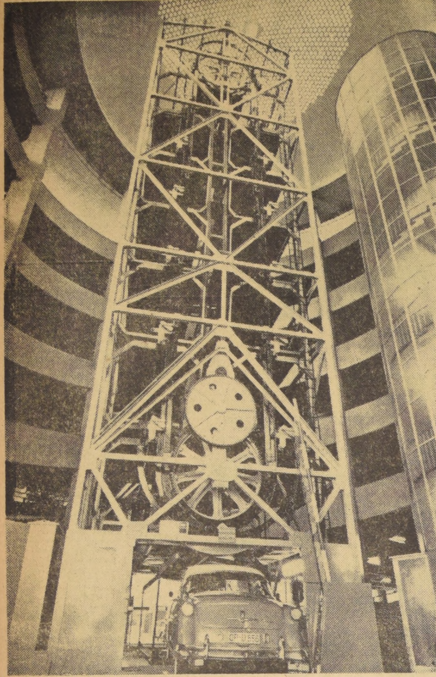
Por todas partes en las grandes ciudades el estacionamiento es un problema. En Colonia se ha buscado remedio en un garaje aéreo en el cual los autos aparecen en el alto. El automovilista entra con el auto en el ascensor, aprieta un botón y sube.
