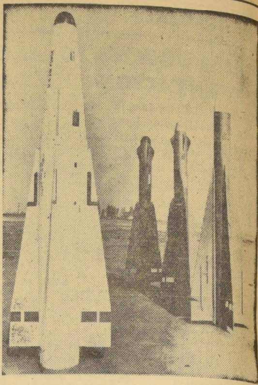
TUCSON, (Arizona).— El aparato blanco de la izquierda es el nuevo cohete nuclear (cohetes) GAR-11, dirigido por radar, primer proyectil guiado de la Fuerza Aérea, con capacidad nuclear. Los tres de la derecha son "hermanos". El cohete tiene siete pies de largo, 11 pulgadas de diámetro y pesa solo poco más de doscientas libras. (Foto UPI).
