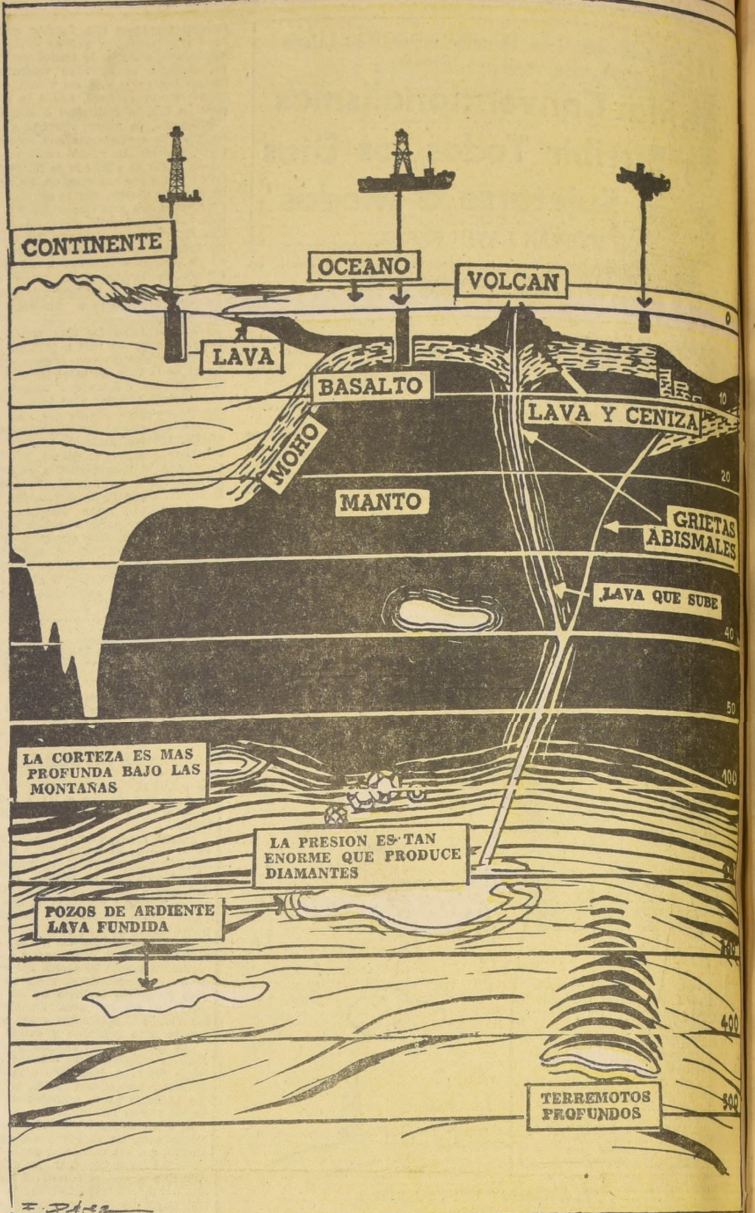
Visión científica del manto de la Tierra, cuna de temblores y cataclismos.
