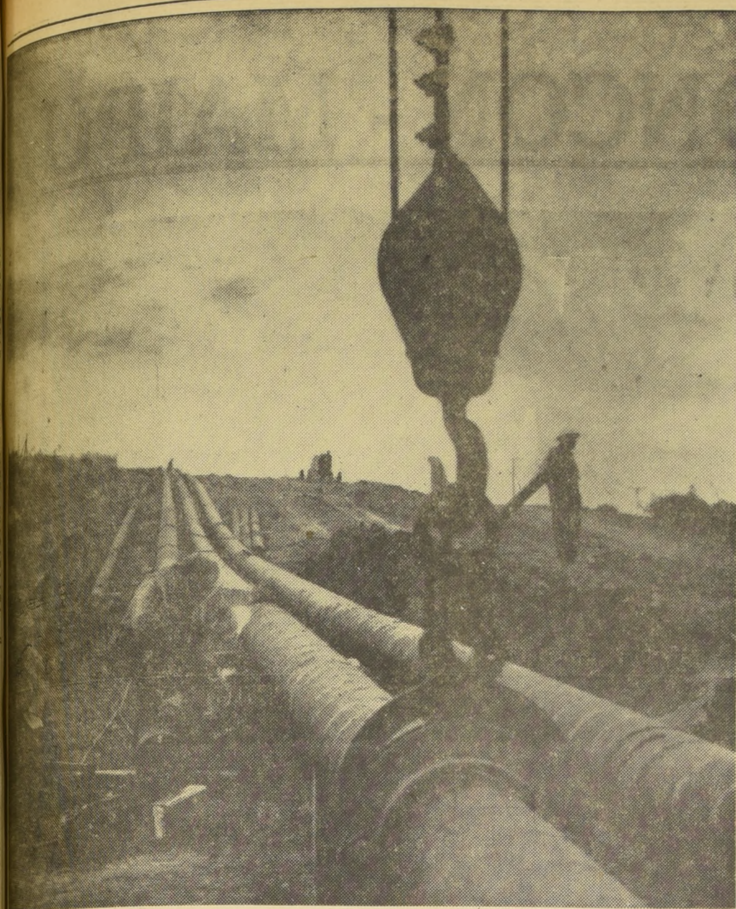
TRABAJO MINUCIOSO Y DIFÍCIL.— Más de veinte mil uniones debieron soldarse en el oleoducto Concón-Santiago, en una labor minuciosa y constante. En el grabado se observa un aspecto de estas faenas, para las cuales se usaron soldaduras INDURA.
