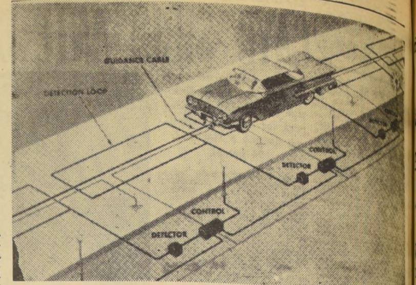
Dibujo esquemático de la carretera electrónica desarrollada por R. C. A. Se pueden observar los cables colocados bajo el pavimento. Este grabado, el circuito de control de la huella luminosa detrás del coche que avanza para advertir a los otros vehículos de su presencia.
