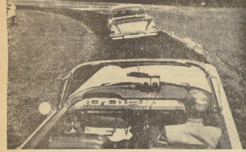
El coche avanza en el Centro de Investigaciones David Sarnoff, en Princeton. Este coche sigue automáticamente la prueba circular y se detiene para evitar una colisión con el coche de prueba que va adelante. Los dos instrumentos colocados en el parabrisas indican la velocidad y la distancia del coche que va adelante, mientras esta información se recibe directamente en los instrumentos que lleva el coche.
