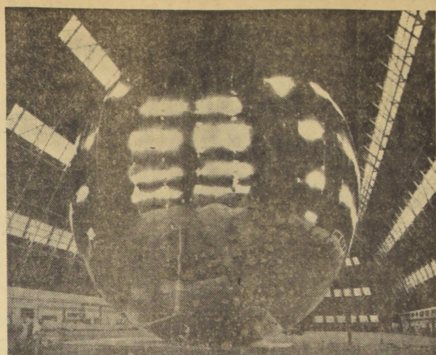
El satélite ECO, de los Estados Unidos, es una enorme esfera de aluminio y material plástico, que refleja las ondas de radio transmitidas desde la Tierra.
