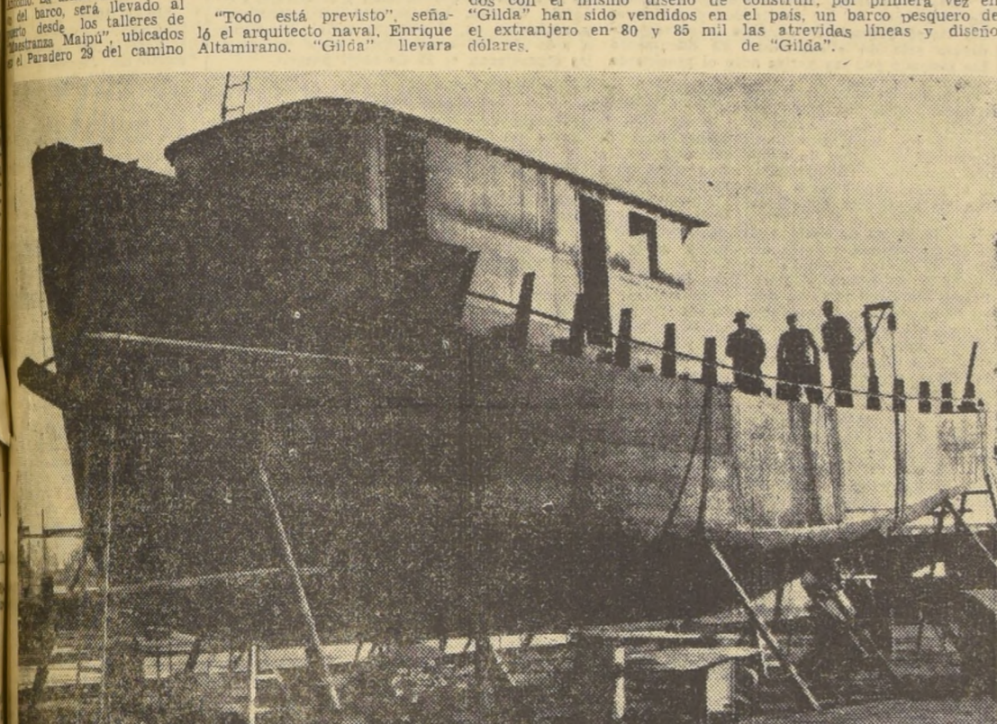
“GILDA” — Este es el primer barco pesquero de acero, construido en Chile. Lo hizo “Maestranza Maipú”, con un equipo de técnicos y obreros de este taller naval de Maipú. Inspeccionan la obra, que quedará totalmente terminada a fines de septiembre.
