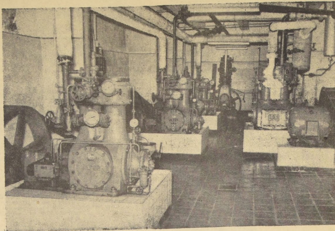
SALA DE MAQUINAS COMPUESTA DE CINCO COMPRESORES CON CAPACIDAD PARA 1.000.000 FRIGORIAS/HORA.
