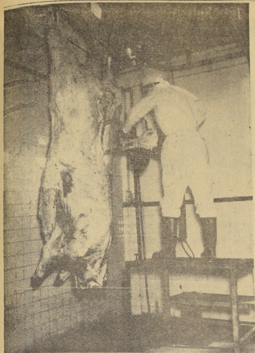
La "sierra eléctrica" en plena labor. La res, sin vísceras, colgada del riel, es llevada hasta la máquina partidora. El operario que se ve en el grabado, en lo alto de una tarima de madera, maneja la sierra comenzando a partirla en dos mitades, de arriba, o sea, desde la cola, ya que ha sido colgada por las patas traseras. Termina de partirla aserrando hasta el cuello a lo largo de toda la columna dorsal, encontrando la mayor resistencia en el tórax y cuello.
