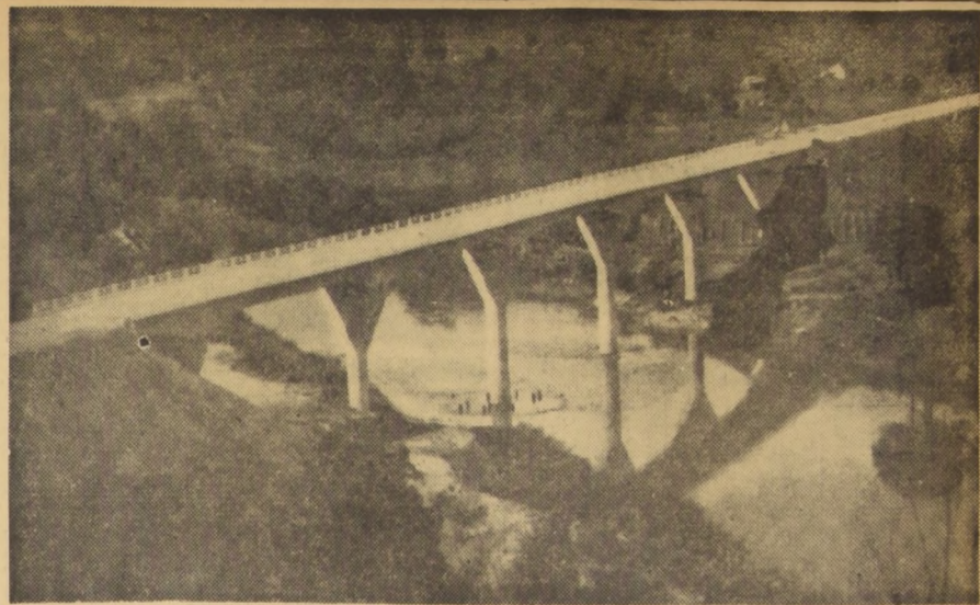
EN EL GRABADO SE PUEDE APRECIAR el extraordinario tipo de construcción adoptado en este puente, apoyado en una sola hilera de pilares, método que se aparta de los sistemas convencionales usados en estos tipos de estructuras.
