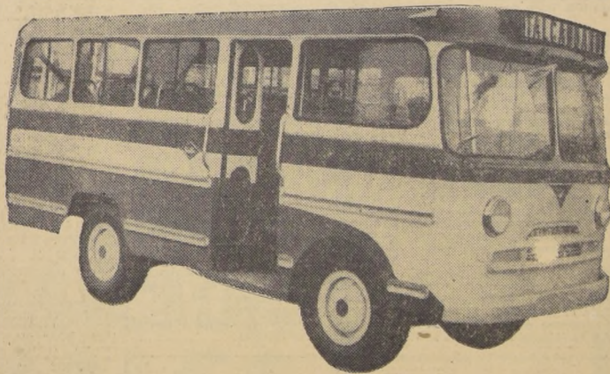
LIEBRE "ISUZU" 17 PASAJEROS — CARROCERIA FRANKLIN, MOTOR DIESEL 52 H. P. — 5 NEUMATICOS, 750 x 15, DE 10 TELAS — CAJA DE CAMBIOS DE 4 VELOCIDADES, SINCRONIZADAS — RENDIMIENTO NORMAL 15 KILOMETROS POR LITRO.
