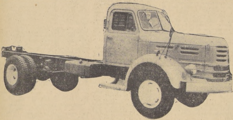
CAMION "ISUZU" 8 TONELADAS, MOTOR DIESEL 190 HP. 7 NEUMATICOS 1000 x 20 DE 14 TELAS — CAJA DE CAMBIOS DE 5 VELOCIDADES SINCRONIZADAS.
