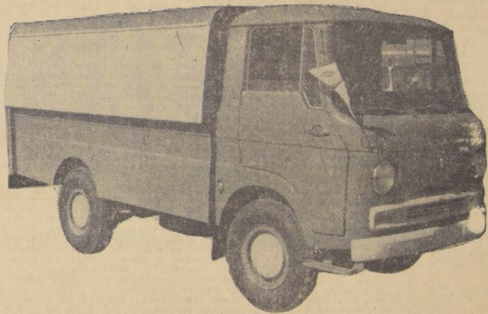
FURGON "ISUZU" 2.000 KILOS DE CARGA UTIL, CARROCERIA FRANKLIN, MOTOR DIESEL 12 H. P., 5 NEUMATICOS 750 x 15 DE 10 TELAS. CAJA DE CAMBIOS DE 4 VELOCIDADES SINCRONIZADAS. RENDIMIENTO NOMAL 15 KILOMETROS POR LITRO.
