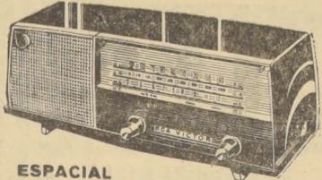
ESPACIAL Funciona con ambas corrientes Ondas Larga y Corta. Antena de Ferrita. Gabinete plástico, ultramoderno. E° 8 AL MES
