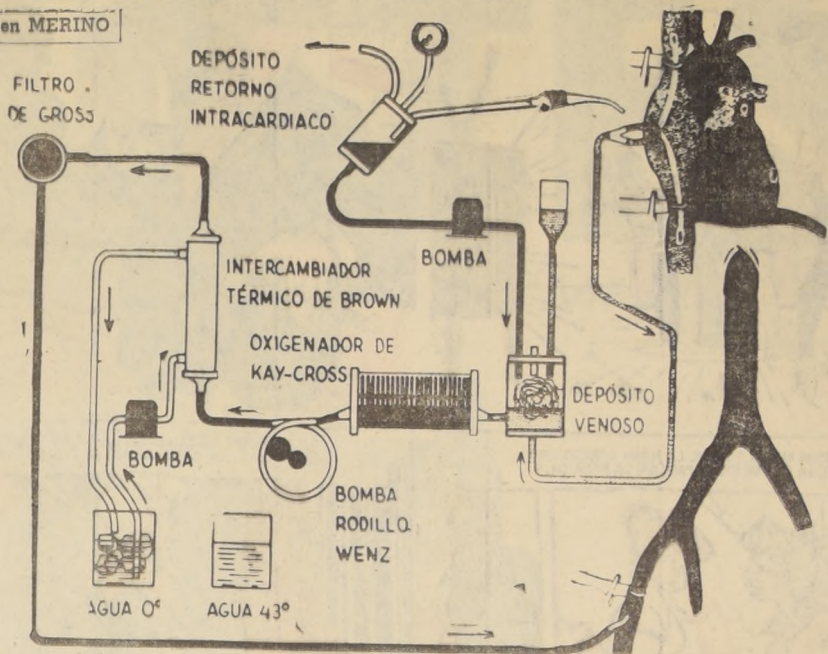
CORAZON-PULMON ARTIFICIAL , mostrado en forma esquemática. A la derecha, arriba, el corazón del enfermo, y los tubos plásticos que entran a la vena cava. Abajo, a la derecha, el tubo plástico que entrega la sangre pura en la arteria femoral. El oxigenador de Kay-Cross permite purificar la sangre que recibe el paciente. El intercambiador térmico de Brown, da la temperatura a la sangre.
