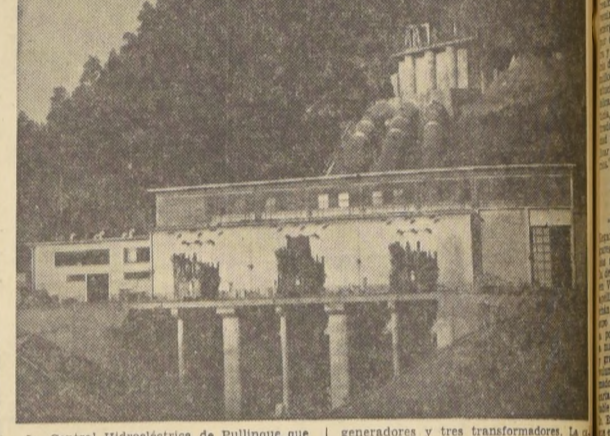
La Central Hidroeléctrica de Pullinque, que fue inaugurada ayer, tiene una potencia instalada de 48.600 KW. Su casa de máquinas está compuesta de tres turbinas, tres generadores y tres transformadores. La casa de máquinas es alimentada por tres tuberías, cuyo diámetro interior de una es de 3 metros y 70 centímetros.
