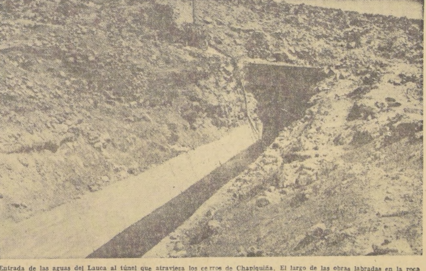
Entrada de las aguas del Lauca al túnel que atraviesa los cerros de Chapiquiña. El largo de las obras labradas en la roca es de cuatro kilómetros y medio.
