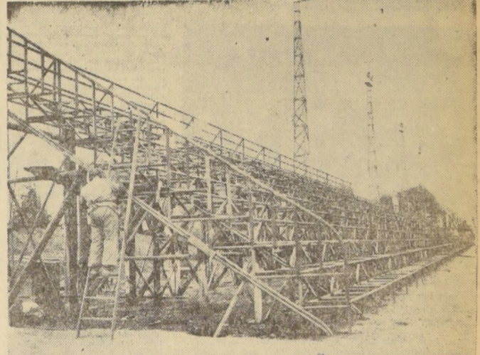
NUEVO ESTADIO — El Club de Deportes San Bernardo Central contará próximamente con un estadio con capacidad para 8 mil personas. En el grabado, puede apreciarse la estructura metálica de las graderías y algunos de los postes de iluminación, que hará de este campo uno de los más cómodos y modernos de que dispone el fútbol.
