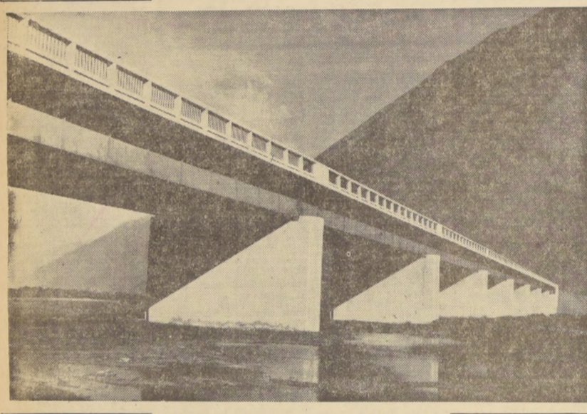
A ciento veinte kilómetros de distancia de Arica y en pleno desierto, levanta su atractiva estructura el Puesto Camarones, de 270 metros de largo y 9,80 metros de ancho, con pasillos laterales para peatones. Siete grandes arcadas, de 31 metros de luz cada una, se levantan sobre el río Camarones. Este puente construido por el Ministerio de Obras Públicas es una de las tantas obras de progreso que se extienden a lo largo del país.
