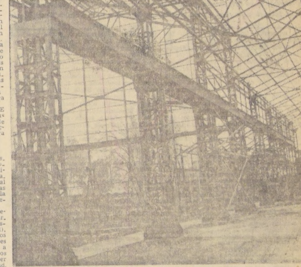
Los planes inmediatos de FAMAE contemplan la construcción de esta sección, cuya armadura metálica se recorta contra el cielo, para instalar en ella su fundición No. 3, con lo que podrá atender sus pedidos siempre en aumento.
