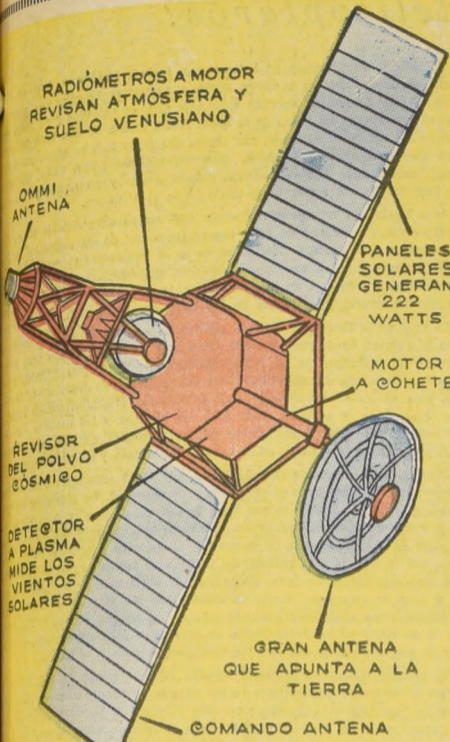
Un esquema del famoso Mariner II, que en estos momentos va en viaje al planeta Venus.
