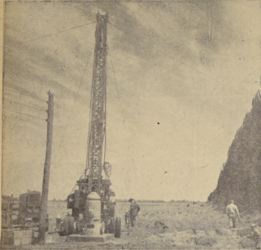
Habilitación de pozo construido por la CORFO, donde se ven la máquina perforadora y un grupo Moto-Bomba para su explotación.
