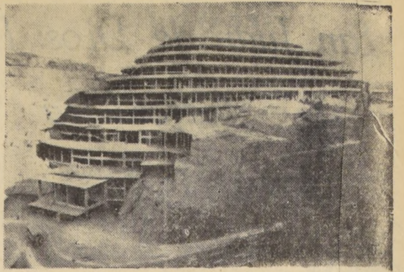
Estado actual de la construcción de "El Helicoide", gigantesca estructura de concreto incrustada en un peñón rocoso.
