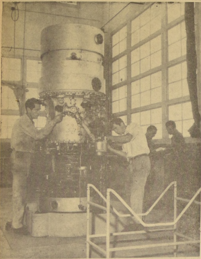
Esta es la primera turbina sometida a recorrida general en los talleres serotécnicos de Aerolíneas Argentinas, ya dotados de los equipos y elementos necesarios. Ha funcionado 3.200 horas en uno de los aviones Comet 4 de la Empresa. En este sector se inicia el desarme total. Luego, cada una de las partes que la componen será sometida a limpieza, inspección, medición, reparación, si es
