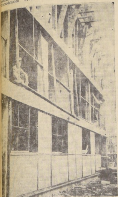
EN LA ESTRUCTURA METÁLICA que enmarca la fachada se apañan los paneles y se colocan las ventanas, ambos prefabricados. La velocidad de la obra es posible advertirla en las diferentes etapas cumplidas en cada piso.
