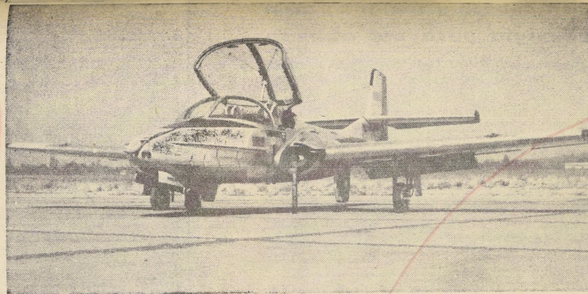
La Escuela de Aviación cuenta con los últimos aviones a reacción fabricados para la instrucción primaria de pilotos en este tipo de máquinas. Estos son los T-37, birreactores que desarrollan en total una potencia de 2.050 libras de empuje y una velocidad de crucero de 240 nudos. En el grabado, sobre la pista de la Escuela un T-37.
