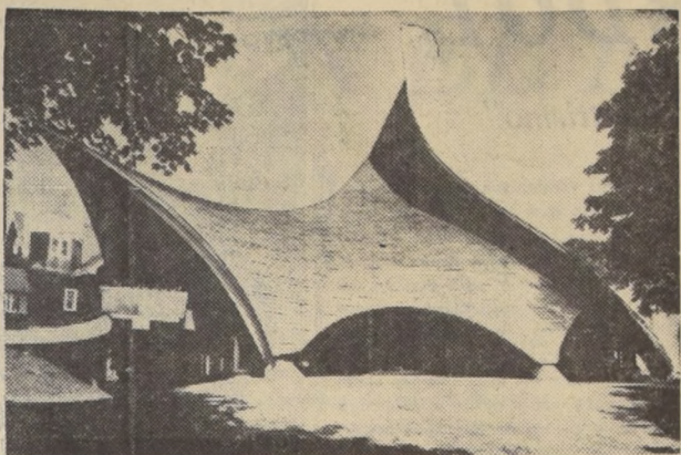
Iglesia Unida de Cristo, Connecticut: Cada viga laminada con cola en el techo de esta Iglesia, está curvada en forma distinta. La superficie del techo es de tejas de madera.
