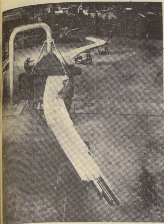
Muchas capas de listones de madera son torcidas con cola para formar una viga construida con exactitud. La viga puede ser producida con cualquier curva, dimensión y resistencia que se deseé para un diseño con espesor de hasta 2.10 metros.
