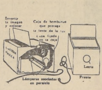
3 Cómo construir un proyector para fotografía en colores
