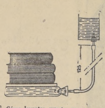
2 Cómo levantar grandes pesos utilizando la presión del agua
