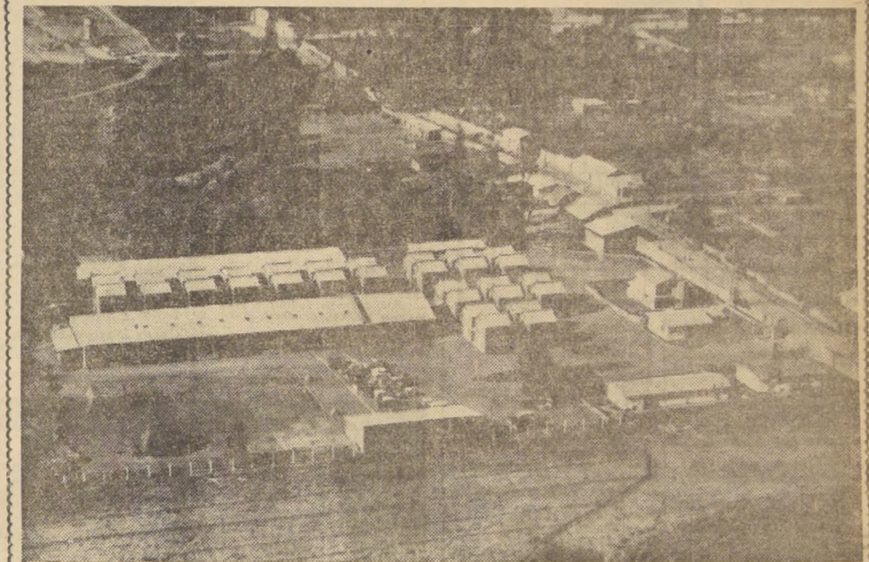
Un magnífico aporte a la agricultura del Norte Chico representa la nueva Planta receptora de tabacos inaugurada por la Compañía Chilena de Tabacos en Salamanca. En el grabado, una vista aérea de la nueva planta industrial.
