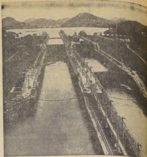
ESLUSA DE MIRAFLORES. SALIDA AL OCEANO PACIFICO DEL CANAL DE PANAMA.
