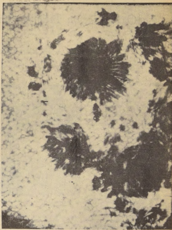
Aspecto de las "manchas" solares fotografiadas desde un satélite artificial
