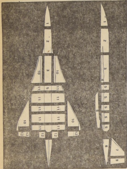
Partes construidas por Francia: 4-ala; 5-parte central del fuselaje; 10-ala delia con bordes de ataque; 11-depositos; 12-postigos, más el acondicionamiento del aire, el equipo de radio y navegación, los circuitos hidráulicos. Partes construidas por los ingleses: 1-cabina del piloto; 2-antefuselaje; 3-fuselaje; 6-reactores; 7-timón; 8-parte trasera del fuselaje; 9-control de la dirección, más la desonorización, el aislamiento térmico, los circuitos eléctricos y de oxígeno.
