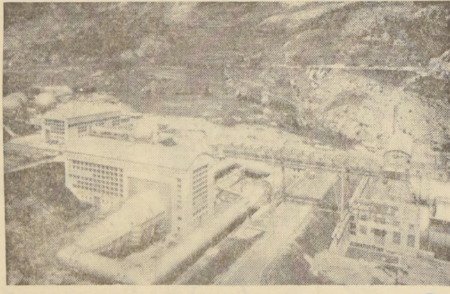
En Modane, esta gigantesca armadura no tiene más que una finalidad: probar minúsculas maquetas. Crea para ello, en este túnel, cubiertas artificiales que se desplazan a 2.500 kilómetros por hora.
