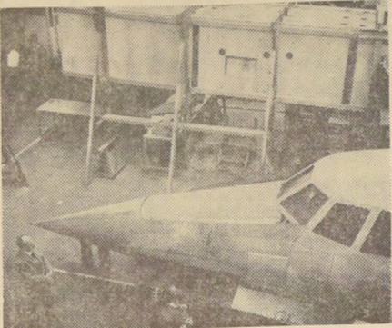
La maqueta de tamaño natural del "Concorde" existe ya en Inglaterra, en madera. Su parabrisa quedará protegido al alcanzar la velocidad supersónica.
