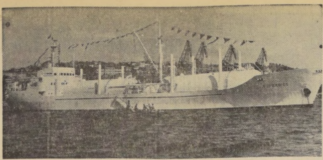
VALPARAISO.—GASERO "COPERNICO". — El gasero "Copérnico" es el segundo barco de este tipo con que cuenta la Marina Mercante Nacional y uno de los cuarenta que existen en el mundo. La mayor característica del barco es la posición horizontal de sus seis estanques almacenadores. Su capacidad de tres mil cuatrocientos metros. En el grabado, el "Copérnico", con su arboladura blanca y chimenea amarilla. Pertenece a la Intercean Gas; empresa propietaria del buque.
