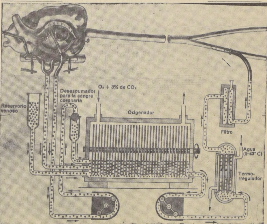
ESTE ES EL ESQUEMA de una máquina corazón-pulmón artificial, que puede reemplazar al corazón durante una intervención quirúrgica de hasta una hora de duración. Entrará en funciones la próxima semana en el Hospital del Salvador. (INFORMACION EN LA PAGINA 14)
