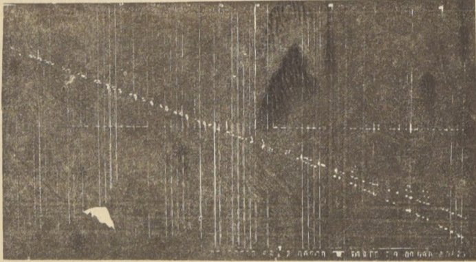
Centelleos entre las dos placas de las cámaras de chispas. Un rayo cósmico que penetra por la parte superior, a la derecha, produce una interacción en un punto.
