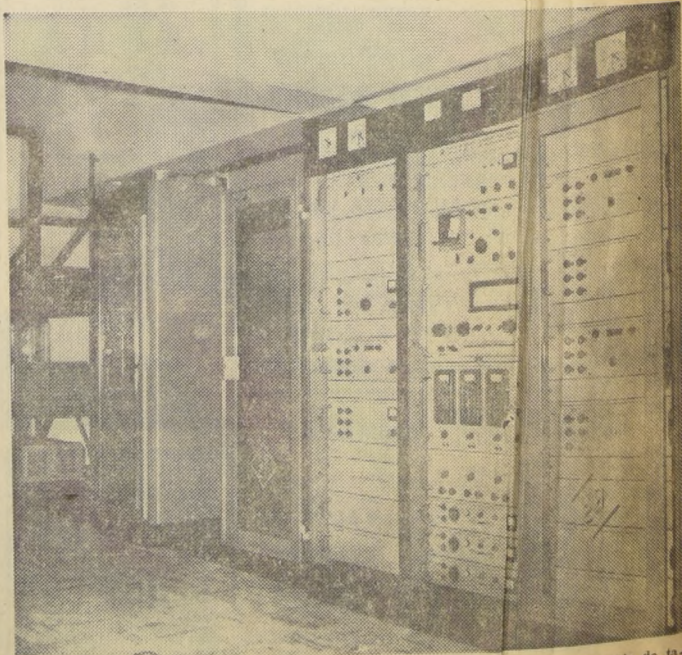
EL OBSERVATORIO Astronómico de la Universidad de Chile, cuenta ahora con un reloj de cuarzo, maravilloso instrumento de precisión que permite una mayor exactitud en la medición del tiempo. El nuevo equipo ha sido recientemente instalado y puesto
